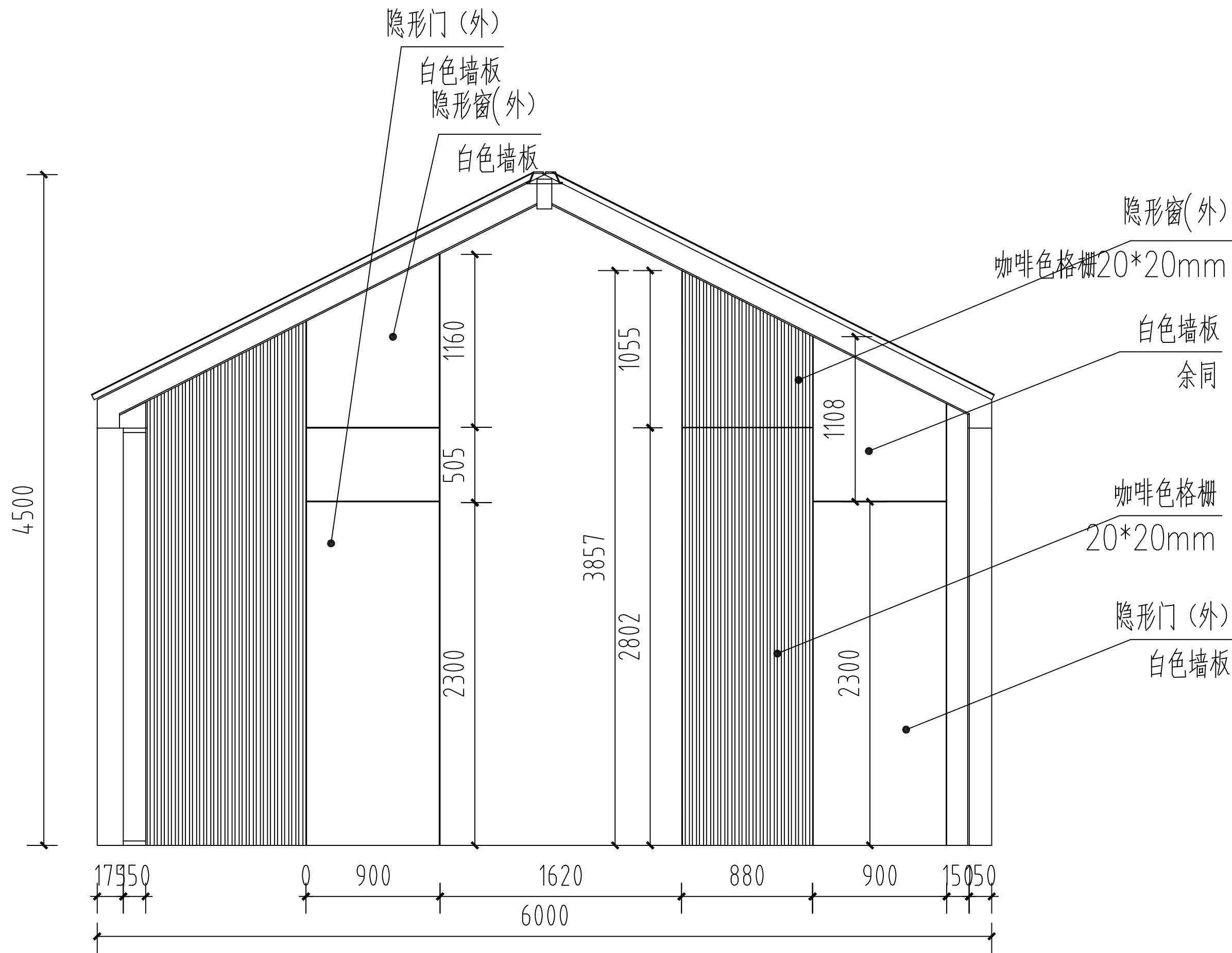
A内视图 1: 25
