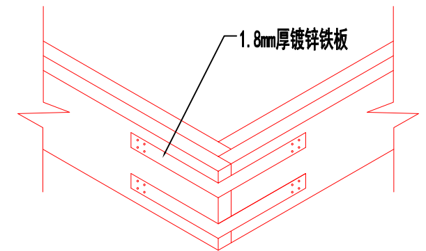
格栅拐角连接详图
