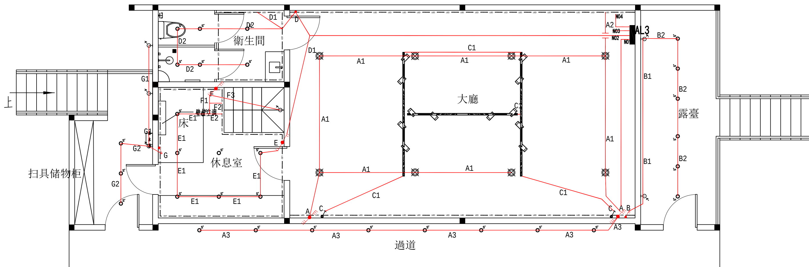
一楼照明平面图 1: 55
