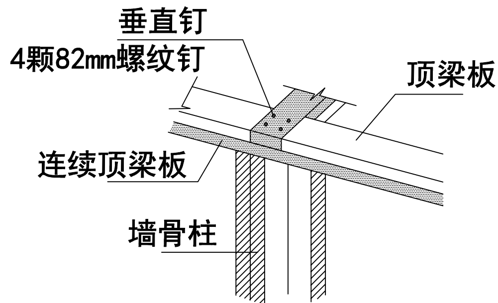
内、外墙体连接详图
