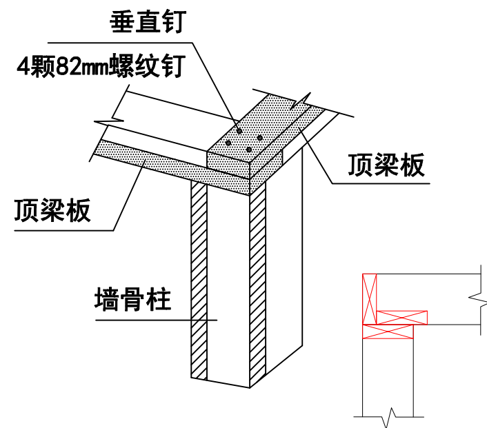
墙体转角连接详图
