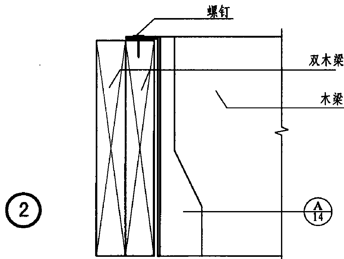
木梁与木梁连接
