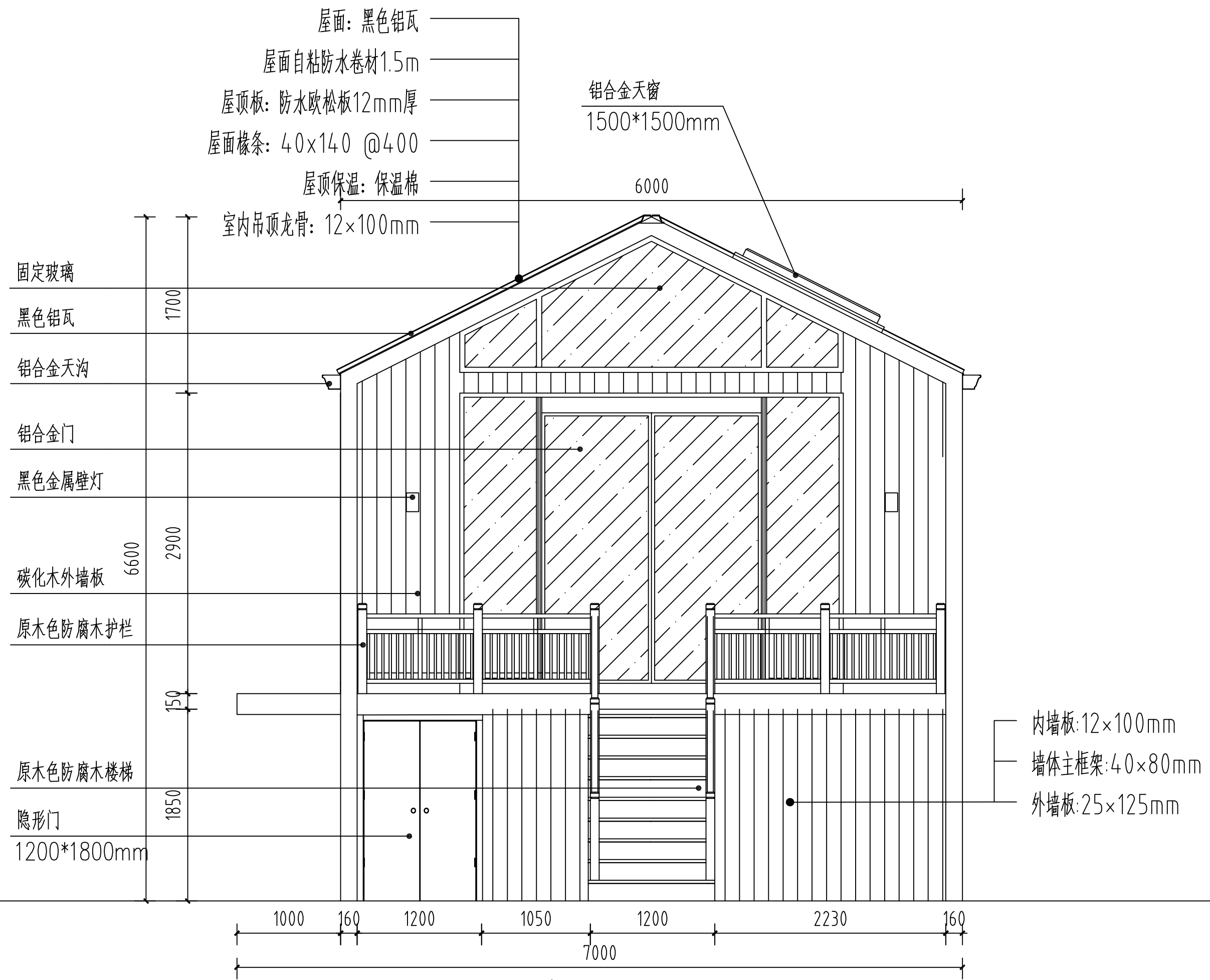
右立面图 1: 35
