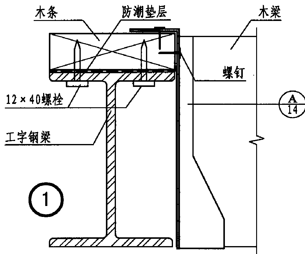
钢梁与木梁连接
