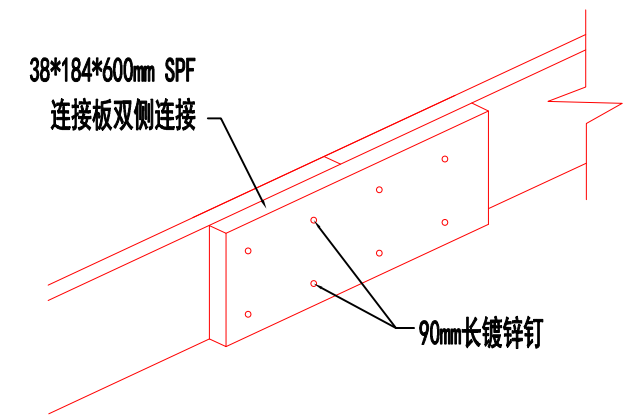
格栅接长连接详图
