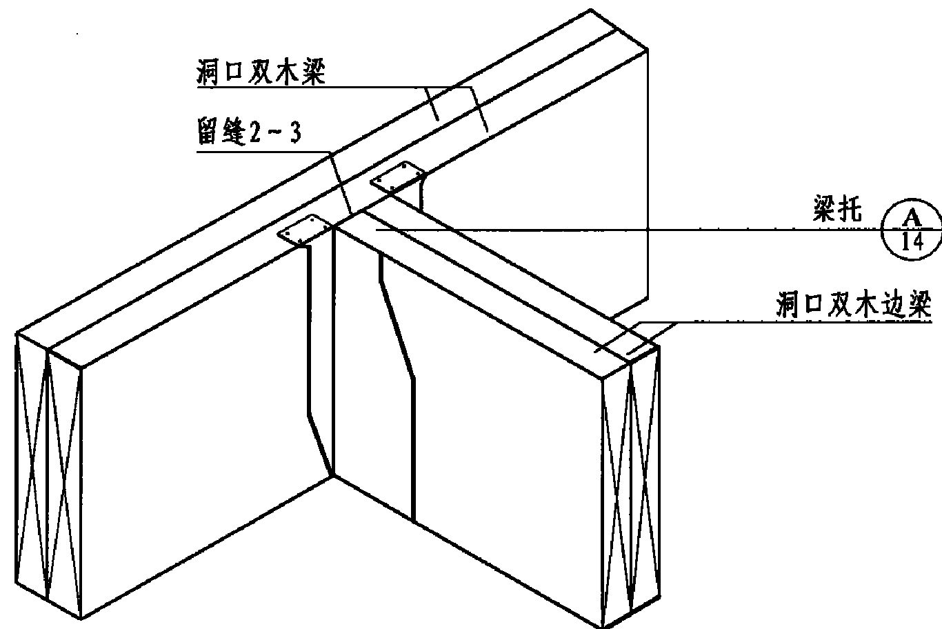
木梁与木梁连接
