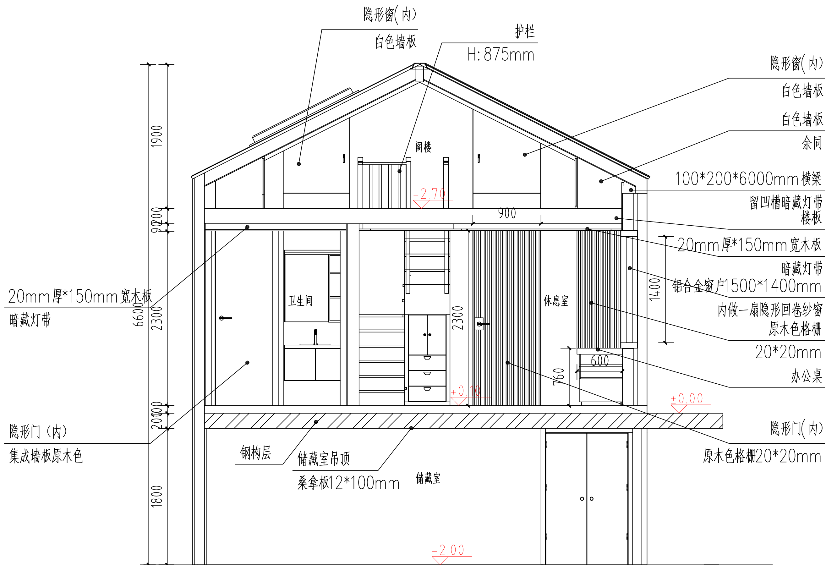
1-1剖面图 1:30
