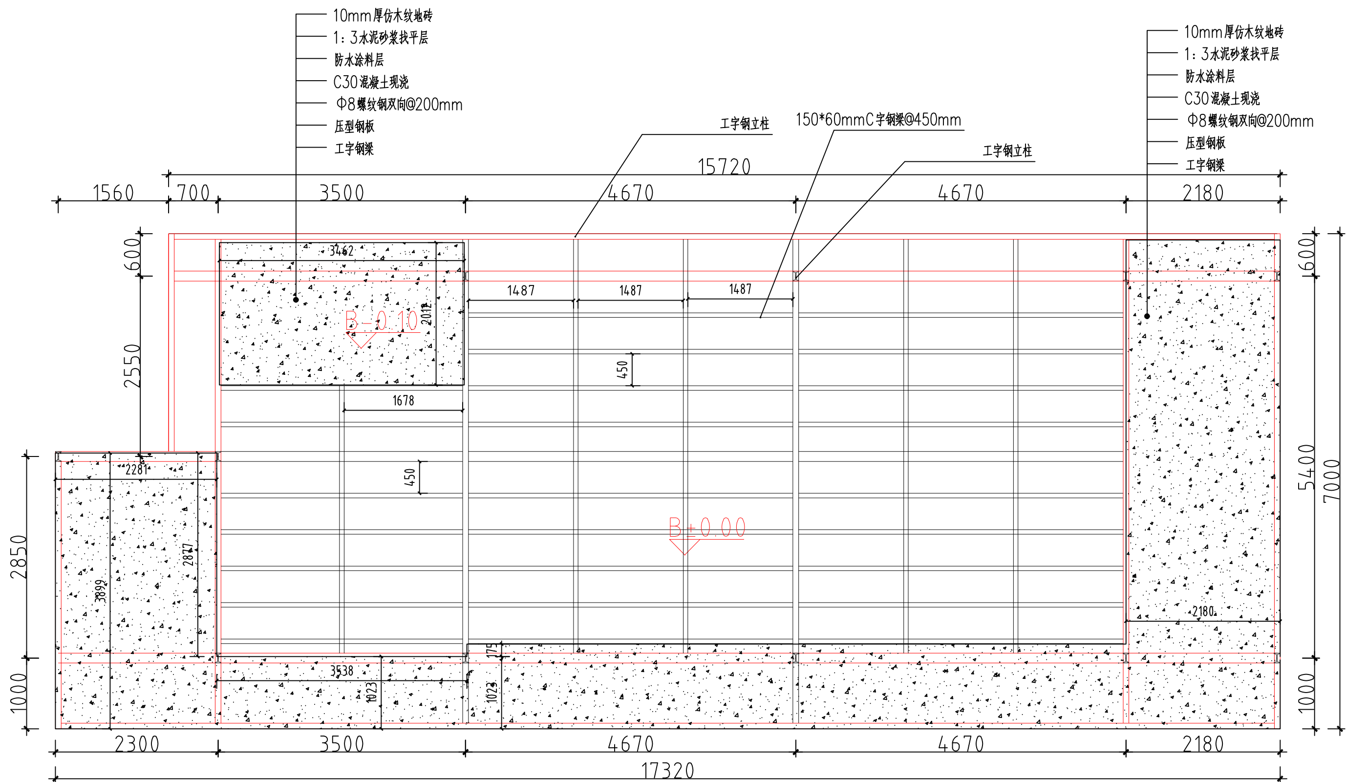
钢结构平面图 1:50
