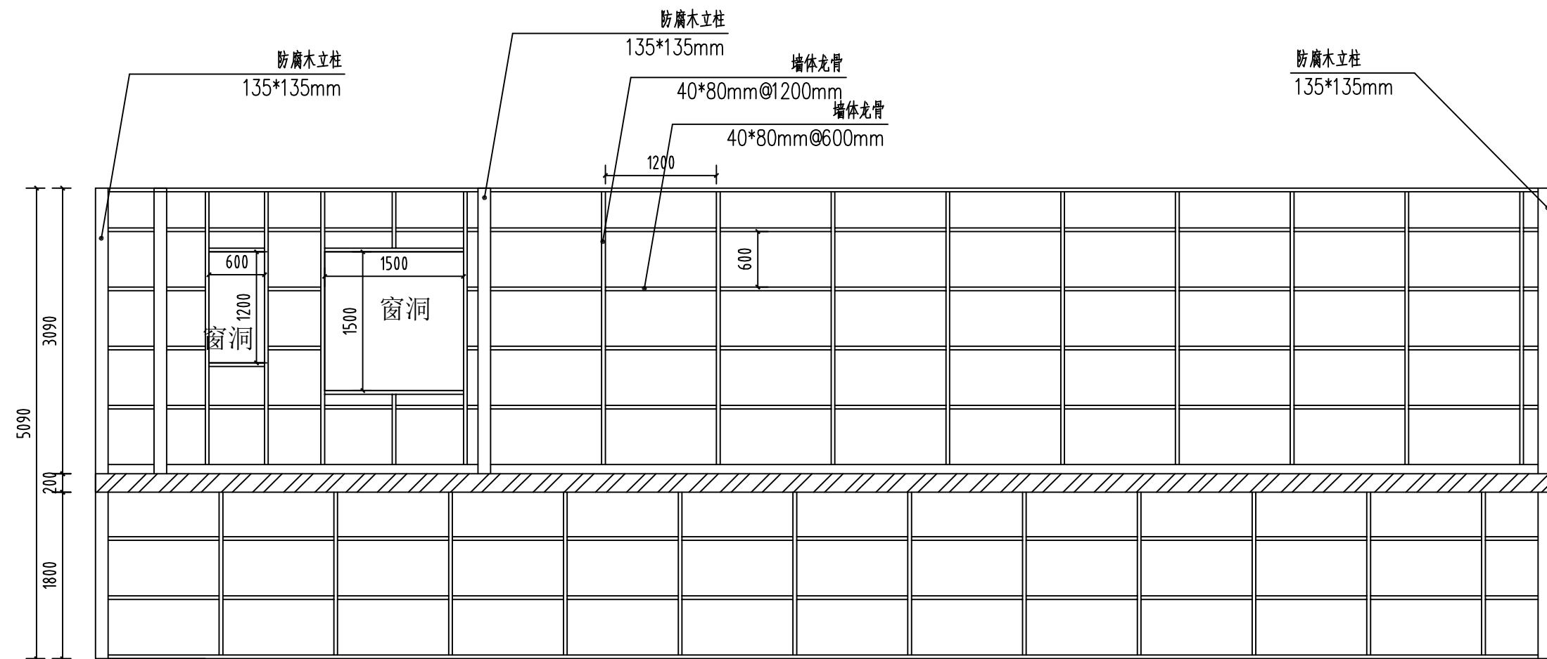
③墙体结构图 1: 30
