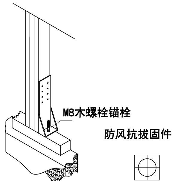
金属防风抗拔连接件大样
