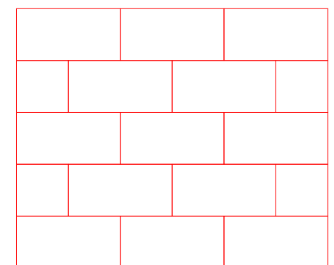
楼面OSB地板排布示意图
