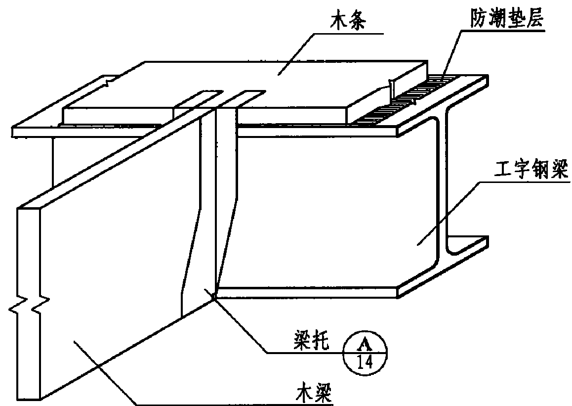
钢梁与木梁连接
