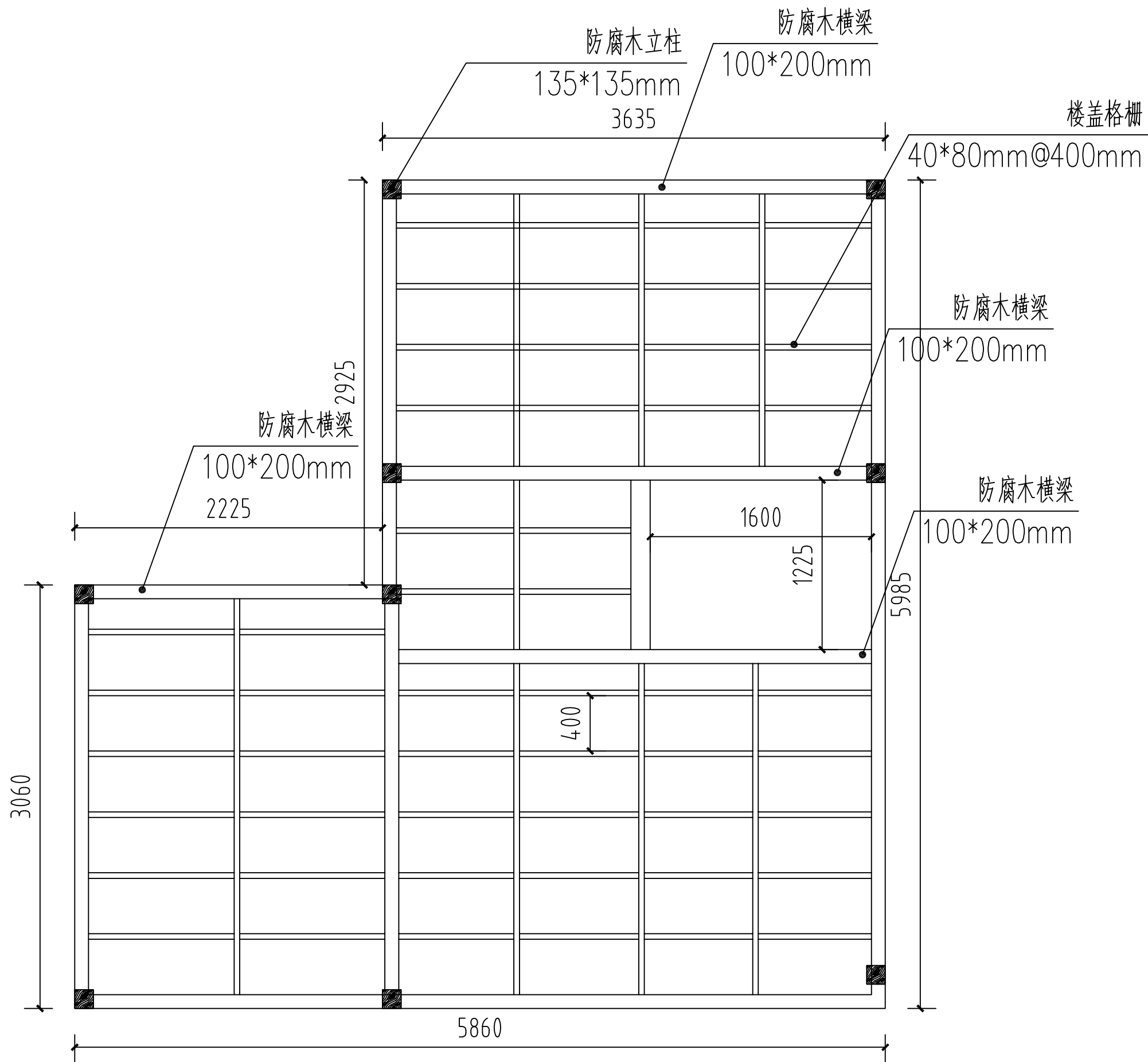
阁楼楼盖格栅龙骨平面图 1: 30
